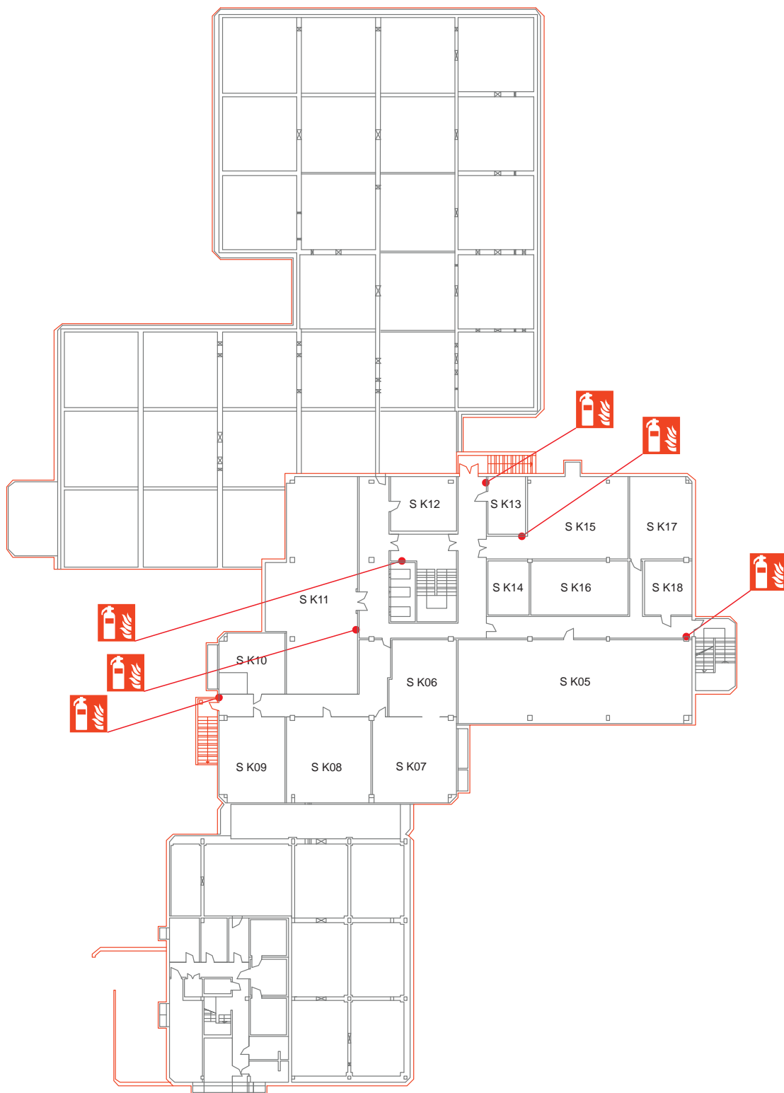
Südgebäude KG.
