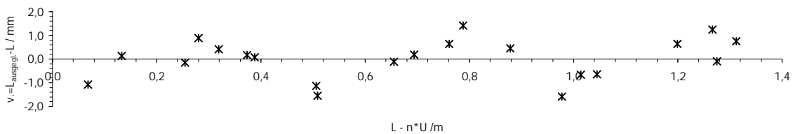
Streckenverbesserungen nach der Ausgleichung bezogen auf Maßstabswelle U
