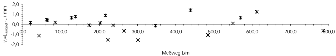
Streckenverbesserungen nach der Ausgleichung
